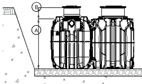
Fig. 17: Profondeur d'excavation / Profondeur d'installation
