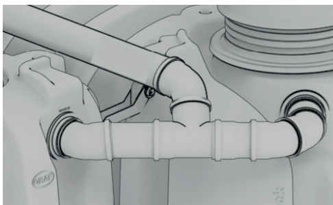
Fig. 35: Raccordements de l'extraction des gaz (ventilation secondaire)
