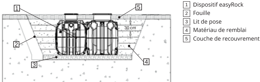
Fig. 11: Schéma d'installation – Vue en coupe du terrain
