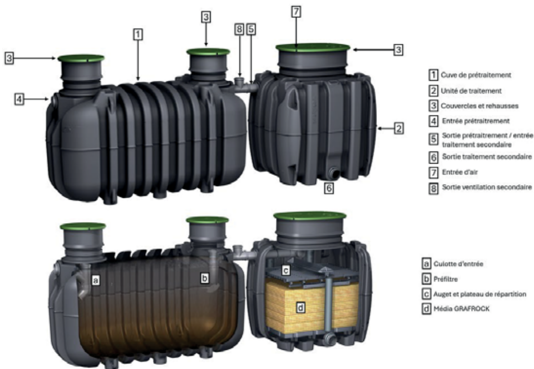
Fig. 2: Aperçu du filtre compact easyRock
