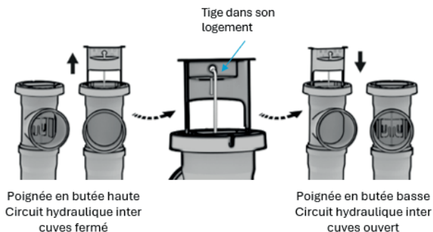
Fig. 54: Manipulation du préfiltre
