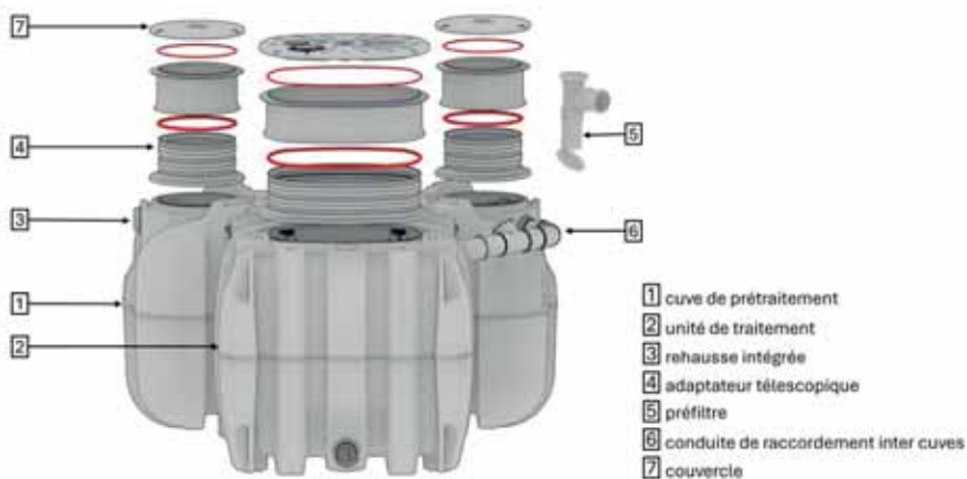
Fig. 6 Matériel livré pour le filtre compact easyRock
