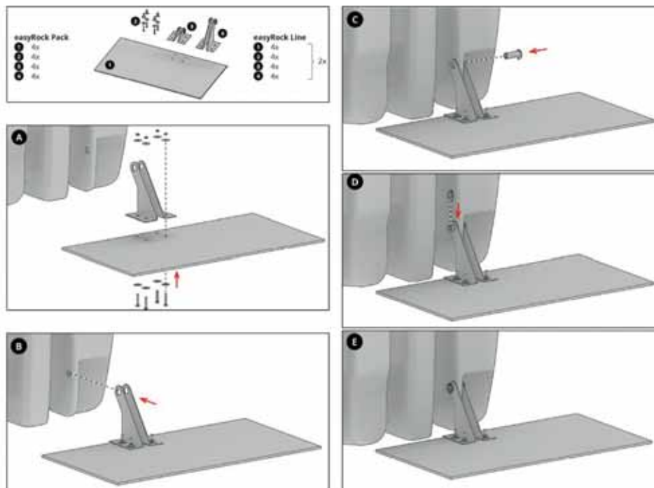
Fig. 47. Montage du kit d'ancrage rapide GRAF
