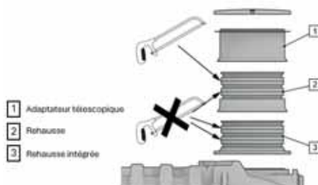
Fig. 22: Adapter les hauteurs
