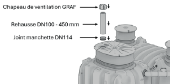
Fig. 45: Installation kit rehausse entrée d'air GRAF
