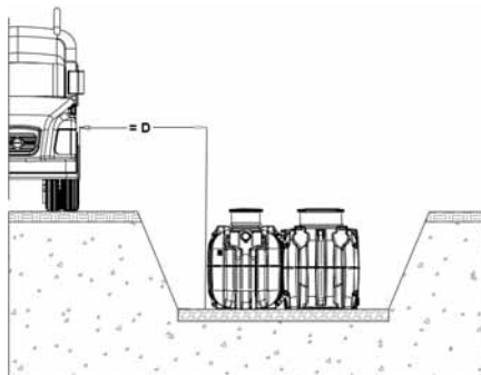
Fig. 14: Écart par rapport aux surfaces de circulation
