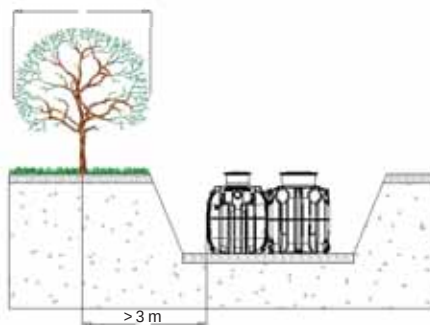
Fig. 12: Distance mini entre système racinaire et cuve
