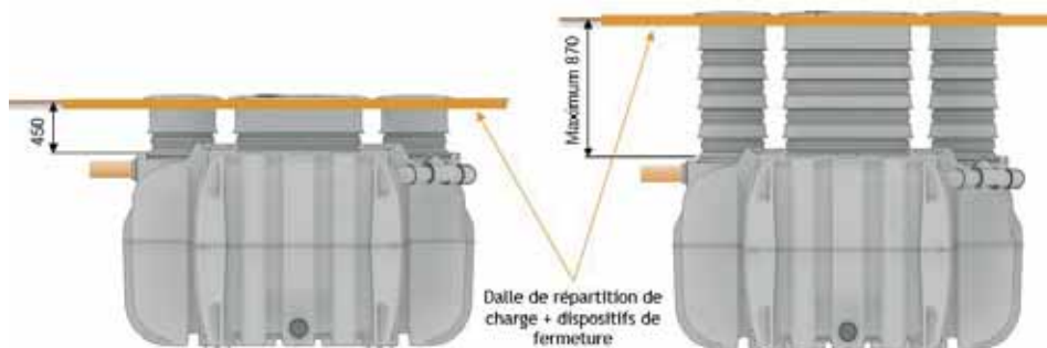
Fig. 23: Schéma d'installation dalle de répartition de charge
