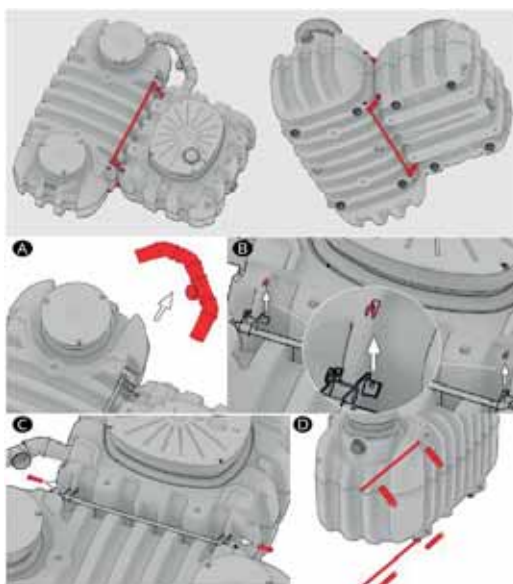
Fig. 46. Désaccouplement des cuves
