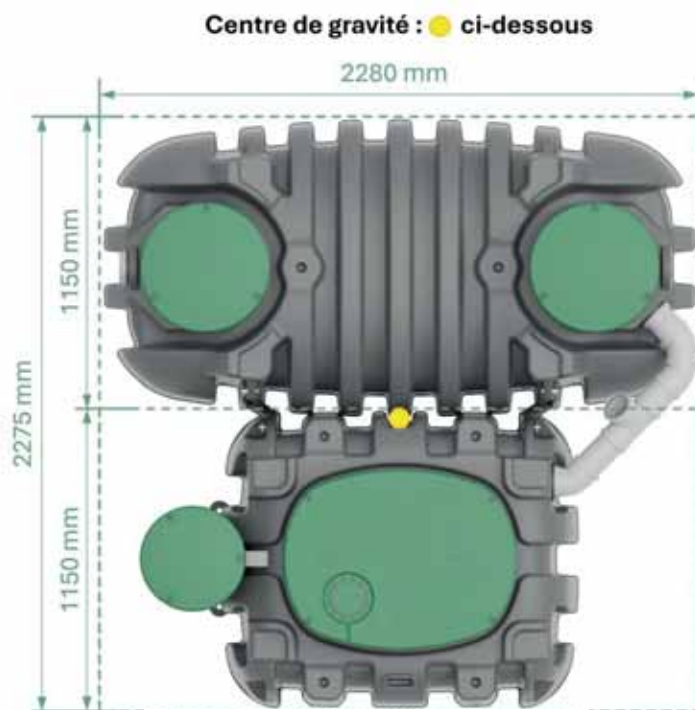
Fig. 7: Position du centre de gravité easyRock 4 EH
