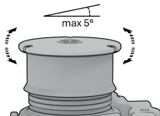
Fig. 37: Adaptateur télescopique
