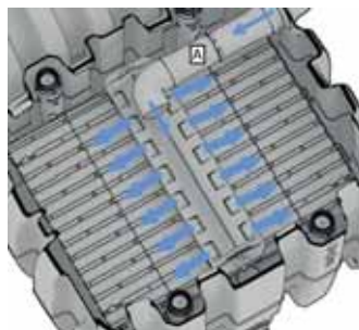
Fig. 40: Arrivée eaux prétraitées et système de répartition
