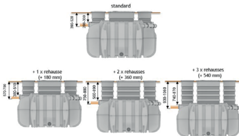
Fig. 21: Hauteurs de recouvrement
