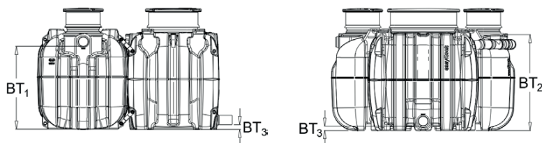
Fig. 20: Cotes de raccords du filtre compact easyRock
