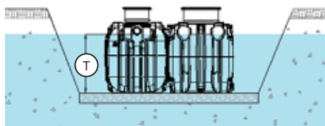
Fig. 19: Profondeur d'immersion maximale
