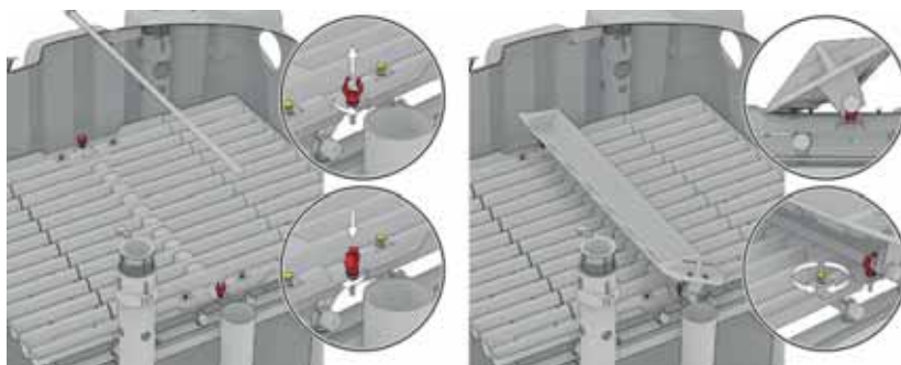
Fig. 58: Ajuster la planéité du système de répartition
