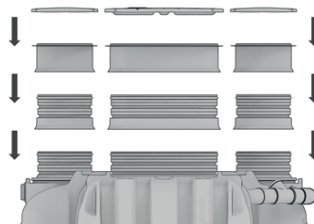
Fig. 36: Mise en place des rehausses intégrées, rehausses et adaptateurs
